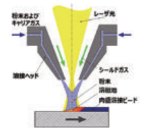
図1 レーザクラディングの概念図
